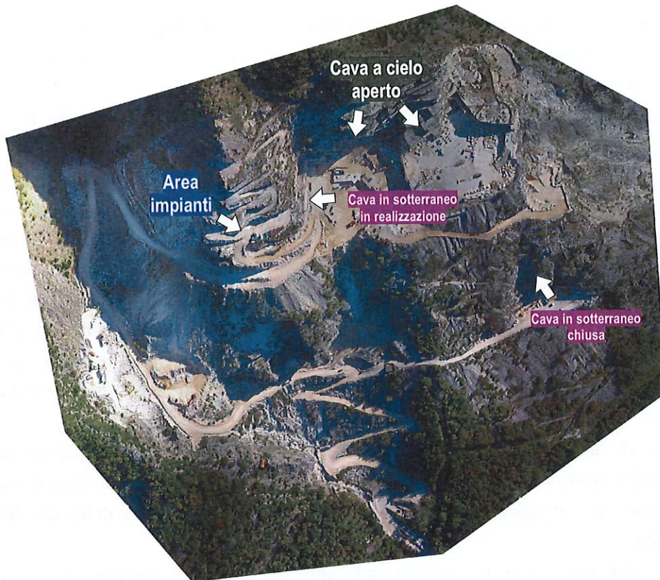
Figura 3 – Ortofoto cava di marmo N.17 RUGGETTA A
