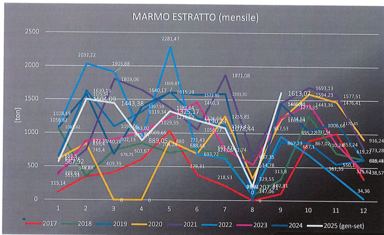
Figura 4 – Marmo estratto su base mensile, dal 2017 a settembre 2025
