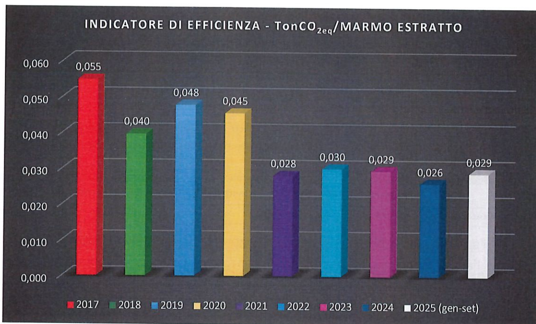
Figura 8 – Indicatore di Efficienza, Emissioni CO 2 in cava (2017 – set 2025).
