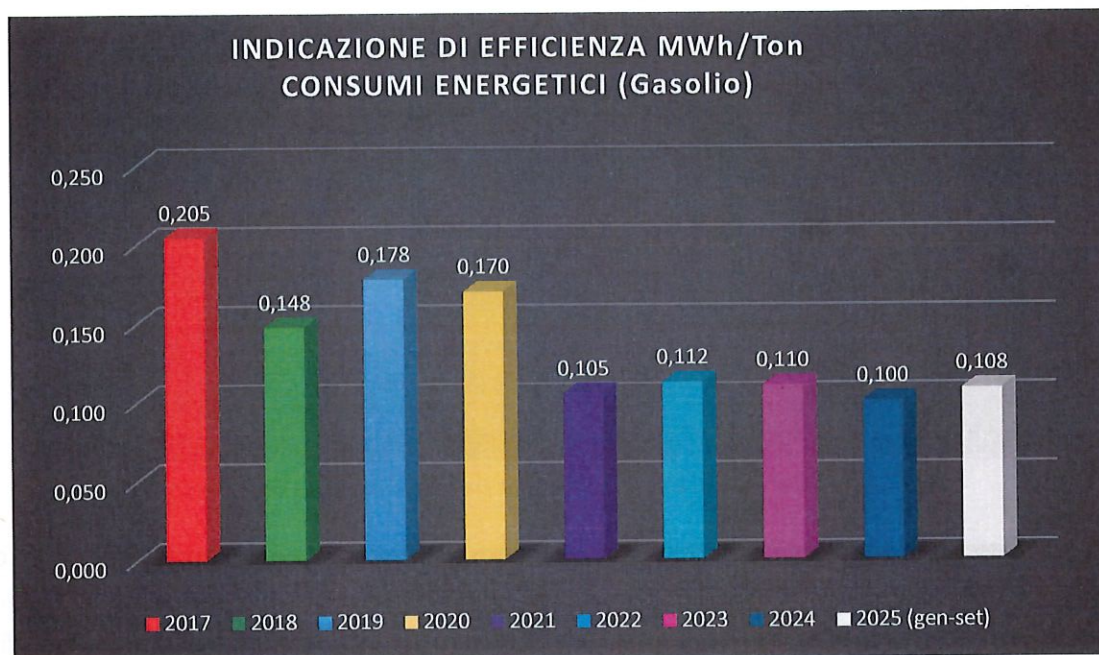
Figura 16 – Indicatore di Efficienza Energetica – Consumo gasolio [MWh] (2017-set2025).
