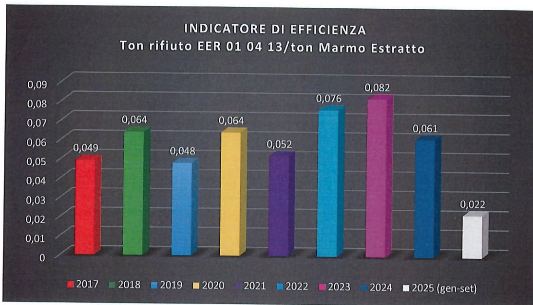
Figura 12 – Indicatore di Efficienza EER 01.04.13 (2017-set2025).
